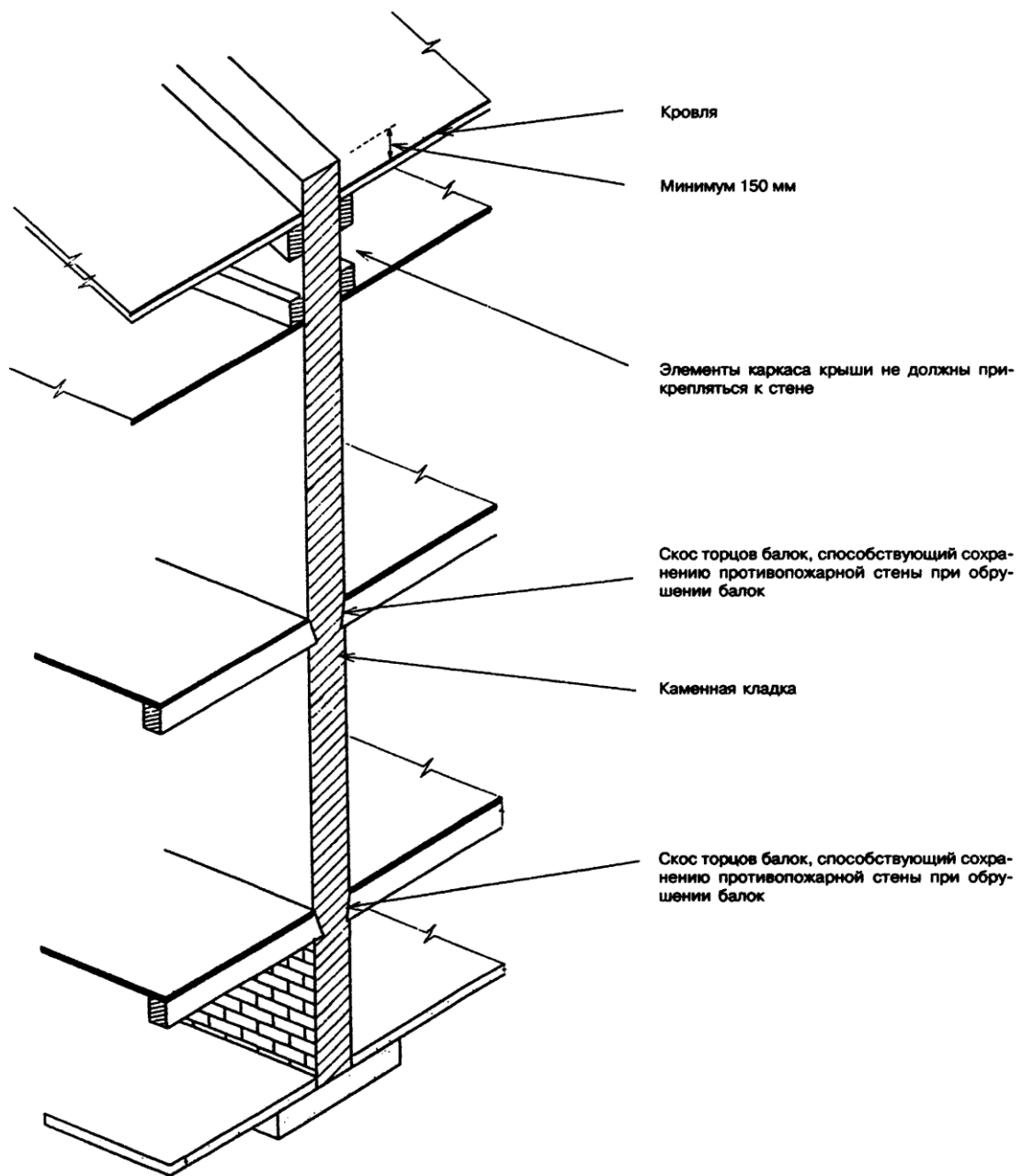
Рисунок 7-5 — Каменная противопожарная стена
