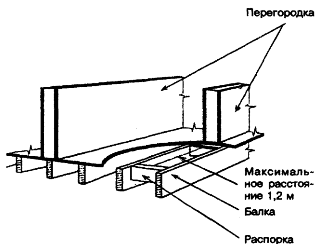
Рисунок 6-13 — Опираение перегородок
