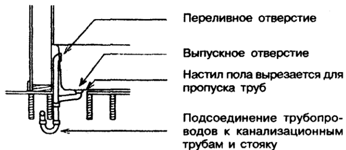
Рисунок 13-6 — Детали установки умывальника и ванны
