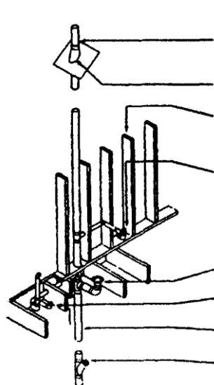
Рисунок 13-8 — Прокладка канализационных труб в каркасе дома
